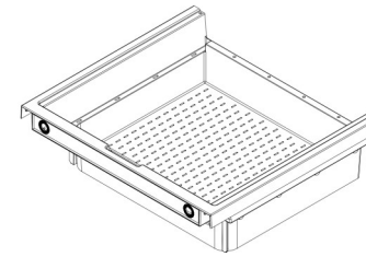
Basisschubkasten NH 170
